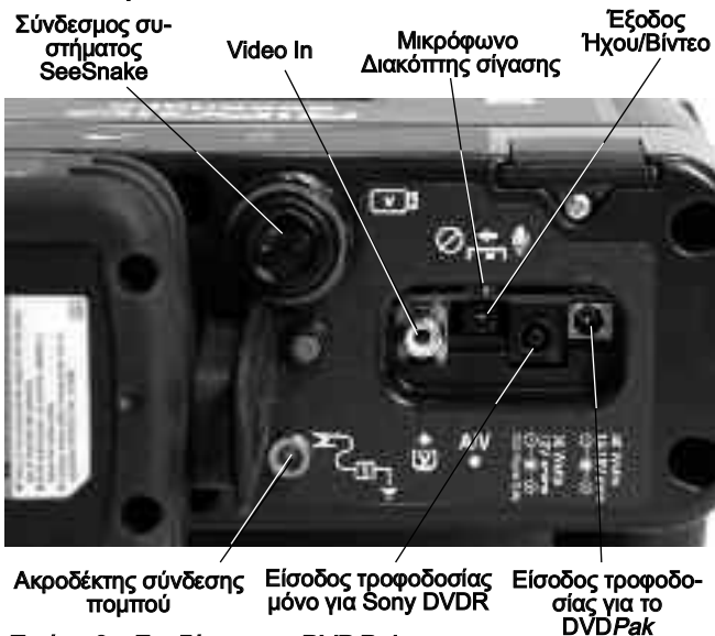
Εικόνα 3 – Συνδέσεις του DVDPak
