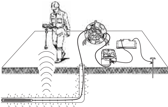
Εικόνα 15 – Ανίχνευση αγωγών της βέργας ώθησης
