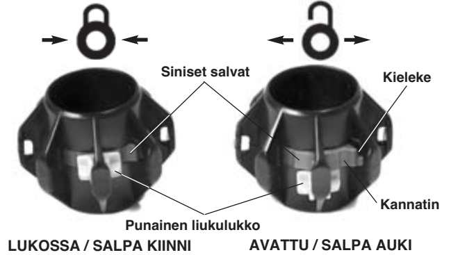
Kuva 15 – Kuulaohjaimen asennus
