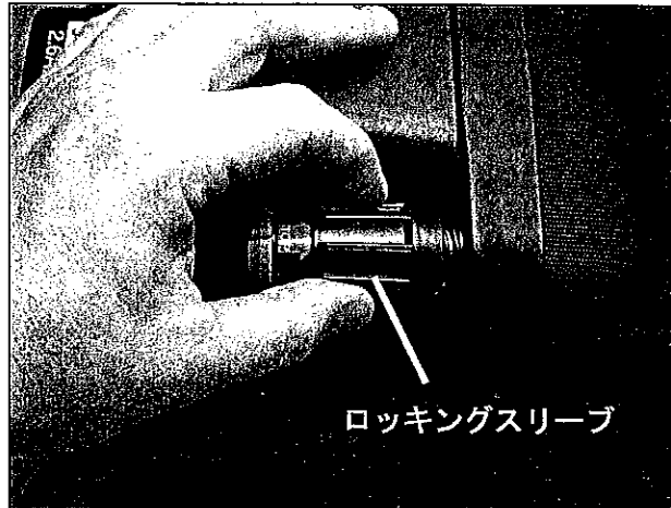
図 12 ロックングスリーブを締める
