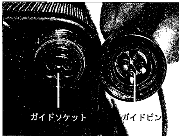
図 13 インターコネクタコードのガイドピン
