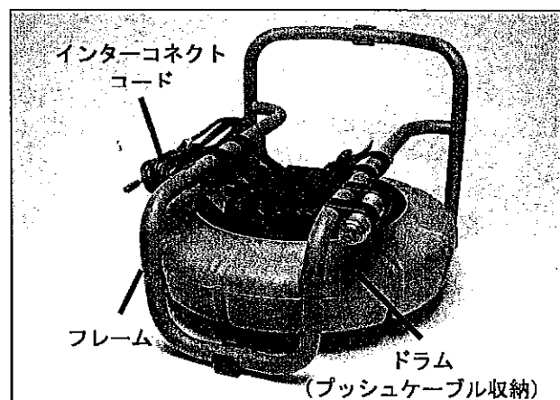
図5 リール/フレーム
