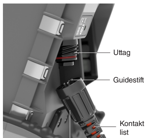
Yttre låshylsa
