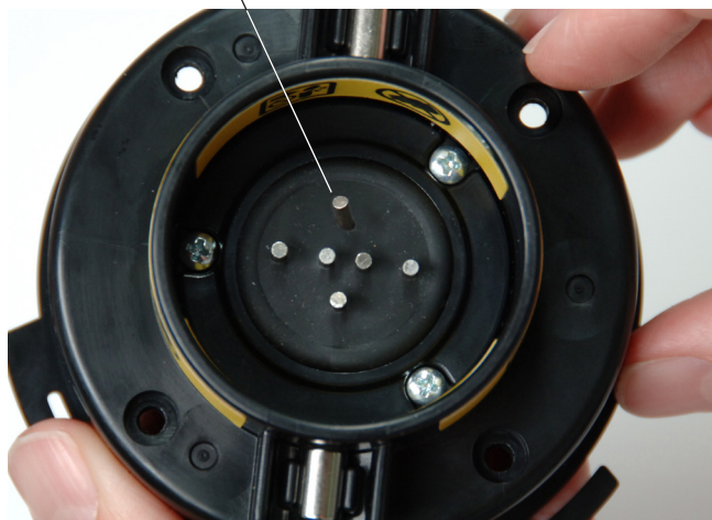
Knækket kontaktstift
