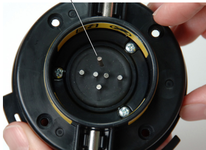
Pin contatto rotto
