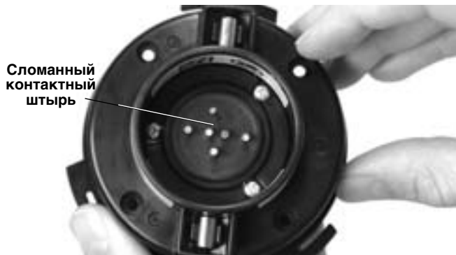
Рис. 7. Сломанный контактный штырь
