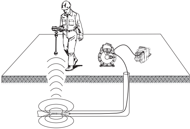
Figura 27 – Localización de la Sonda del microReel
