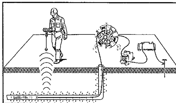
図 11 プッシュロッドによる経路トレース
