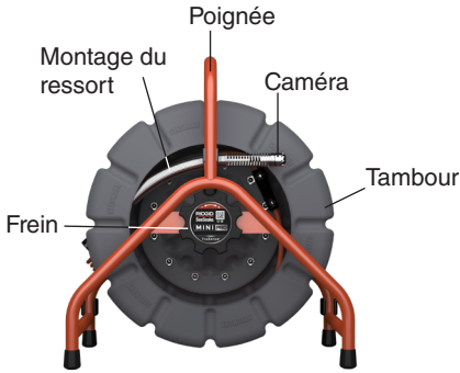
Câble de poussée
