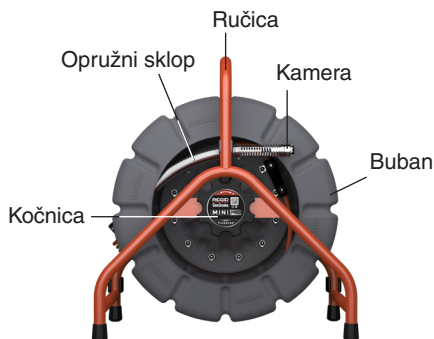
Potisni kabel
